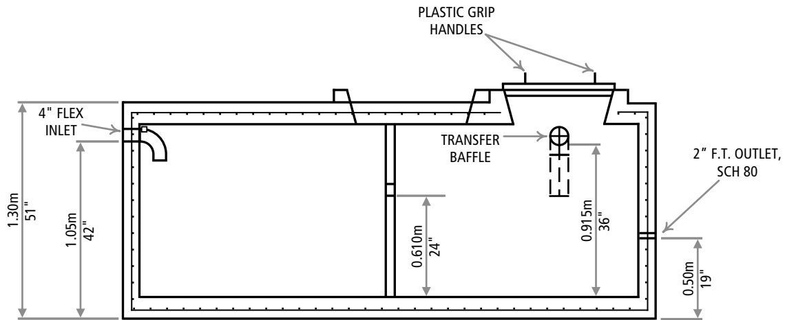
SECTION A-A
